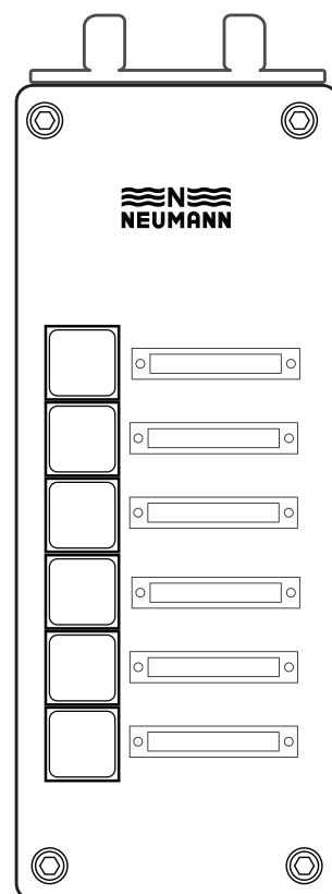
WFAK Zusatzgehäuse, gelb 6 Leuchtdrucktasten Art.-Nr. 1 977 4
