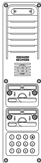
WFD Wetterfeste Digitale U p0 Sprechstelle, 2 Doppelknebel + Wahltastatur Art.-Nr. 1 632 2
