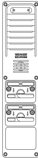
WFD Wetterfeste Digitale U p0 Sprechstelle, 2 Doppelknebel Art.-Nr. 1 639 9 Mit 25W Zusatzverstärker Art.-Nr. 1 636 6
