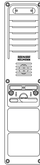
WFD Wetterfeste Digitale U p0 Sprechstelle, 1 Doppelknebel Art.-Nr. 1 638 8 Mit 25W Zusatzverstärker Art.-Nr. 1 635 5
